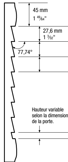
PROFIL DE COUPE VERTICAL
