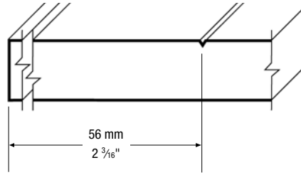
ALIGNEMENT ENTRE PORTES ET TIROIRS JUXTAPOSÉS
