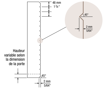
PROFIL DE COUPE VERTICAL
